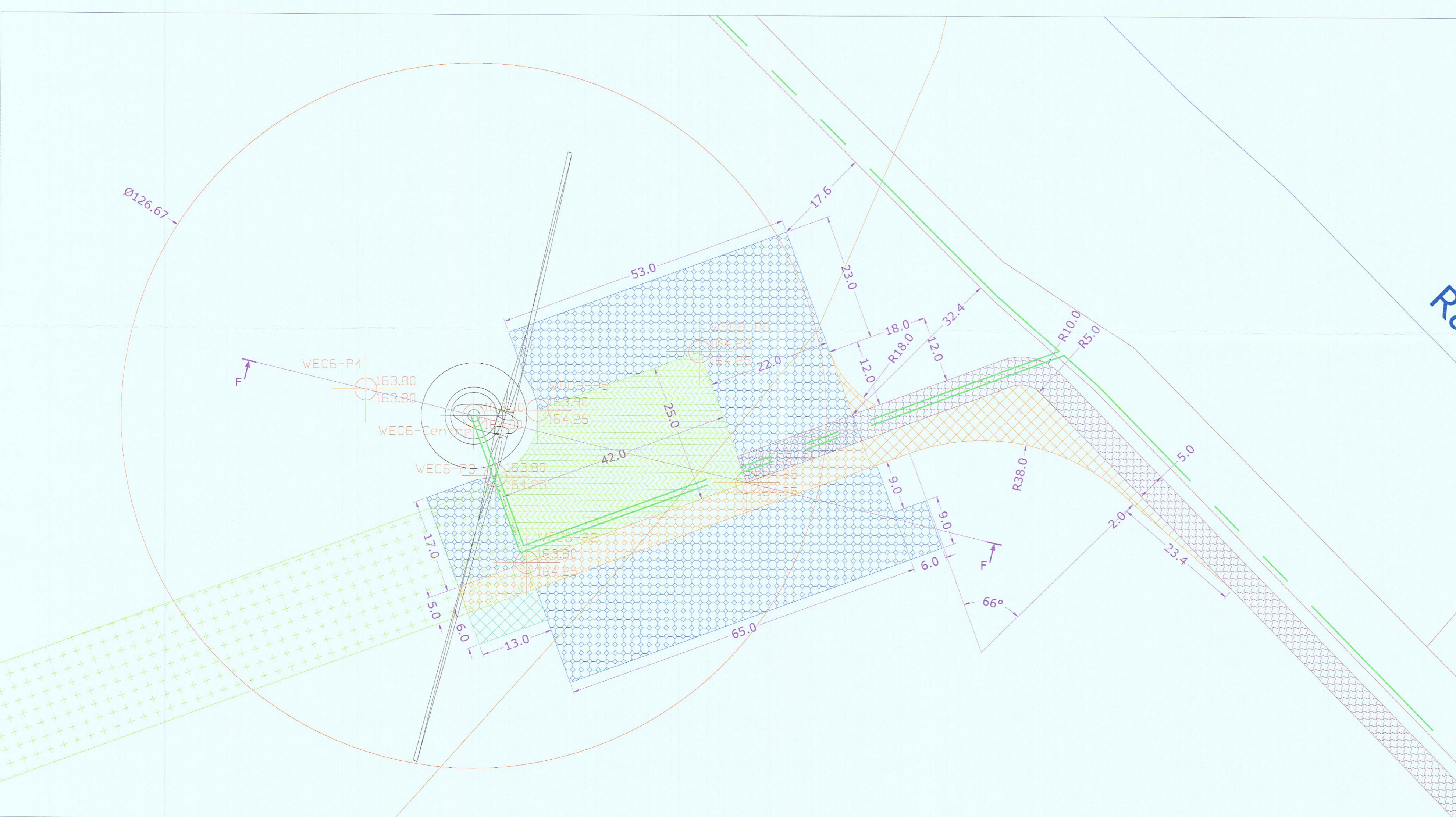
DETAIL EOLIENNE 6 (1/500)
